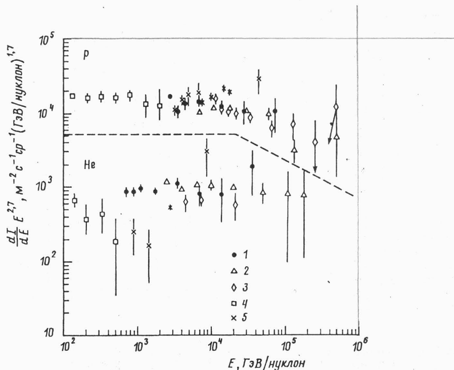
Рис. 1. Дифференциальные энергетические спектры протонов и ядер He. Точки 1 — данные настоящей работы, 2 — [3], 3 — [4], 4 — [10], 5 — [12]
