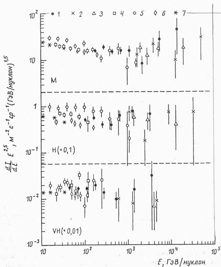
Рис. 2. Дифференциальные энергетические спектры ядер групп М, Н и Н. Точки 1 — данные настоящей работы, 2 — [3], 3 — [4], 4 — [13], 5 — [14], 6 — [15], 7 — [16]
