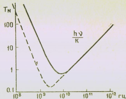
Рис. 1. Спектр шумов вне пределов земной атмосферы: — в направлении на центр, - - - - в направлении на полюс Галактики.
