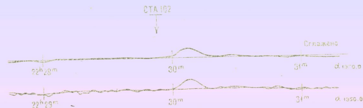
Рис. 1б. Кривая прохождения источника СТА-102 (внизу). Вверху — сглаженная кривая на интервалах 1' .
