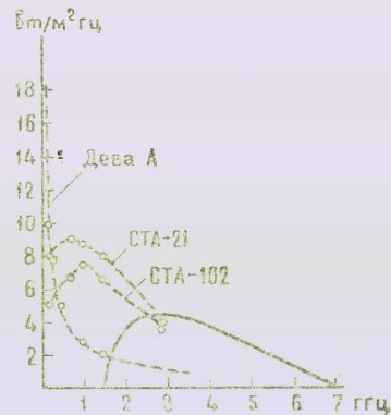
Рис. 2. ———— ожидаемый спектр излучения радиопередатчиков суперцивилизаций; — — — — спектр радиоисточников СТА-21 и СТА-102, подозреваемых в качестве искусственных, и спектр радиогалактики Дева А.
