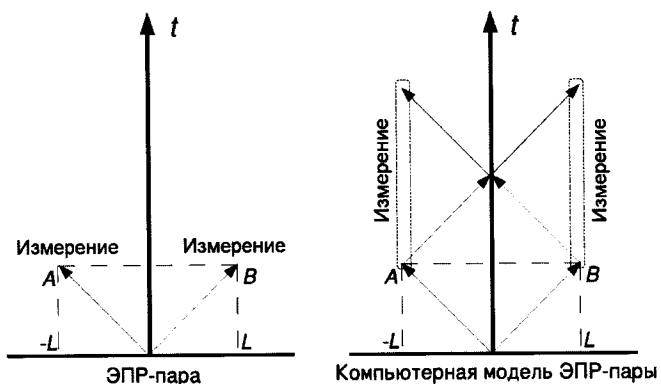
Рис. 4. Пространственно-временные диаграммы измерений спинов для реальной ЭПР-пары и для компьютерной системы, симулирующей измерения
