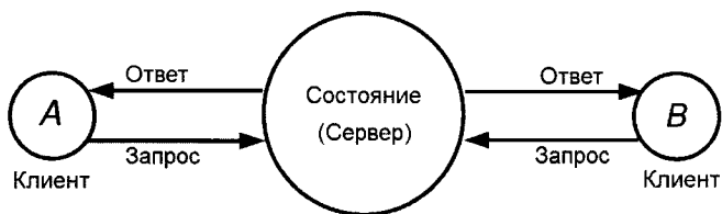
Рис. 2. Структура программы, симулирующей измерение спинов над скоррелированной ЭПР-парой
