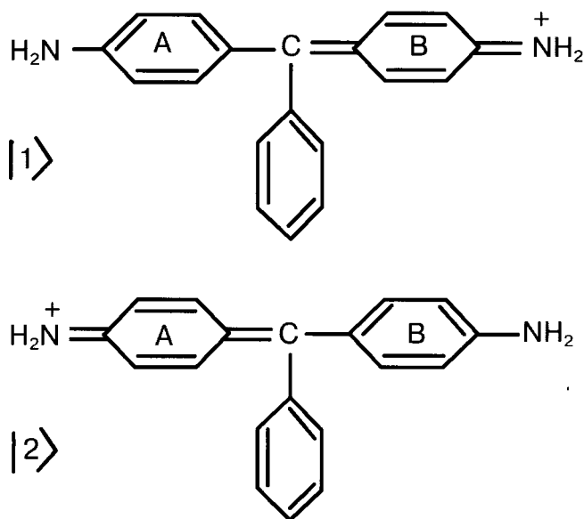
Рис. 1. Две конформации (два базисных состояния) молекулы красителя фуксина
