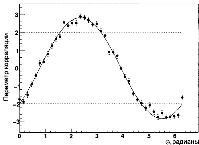
Рис. 3. Результат симуляции поведения ЭПР-пары компьютерной программой. Точки с ошибками — результат симуляции, сплошная кривая — предсказание квантовой механики, горизонтальные штриховые прямые — ограничения на значения корреляции, налагаемые неравенствами Белла
